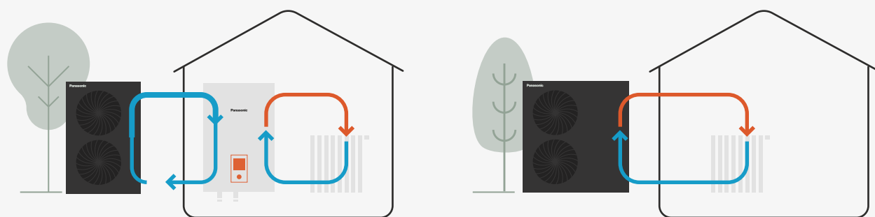
Rys. 5 Różnica pomiędzy pompa ciepła typu split a monoblok
